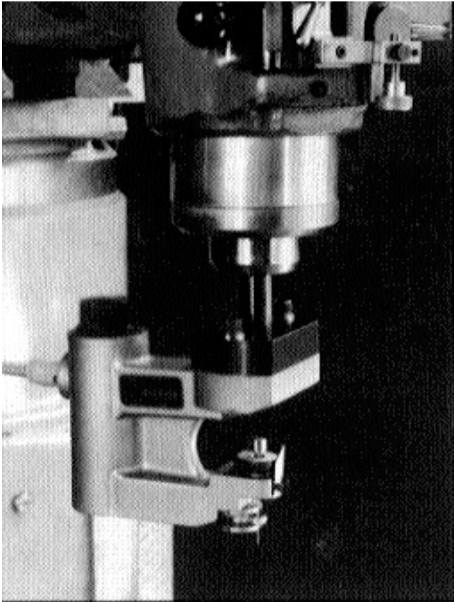
ブリッジポート社のミリングマシンに取り付けたModel 2000
